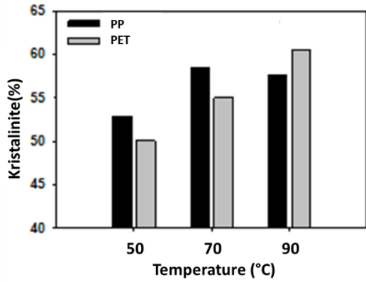
Şekil 1. PP ve PET'in kristalinitesinin karşılaştırması
